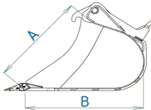
Tieflöffel Serie 2
