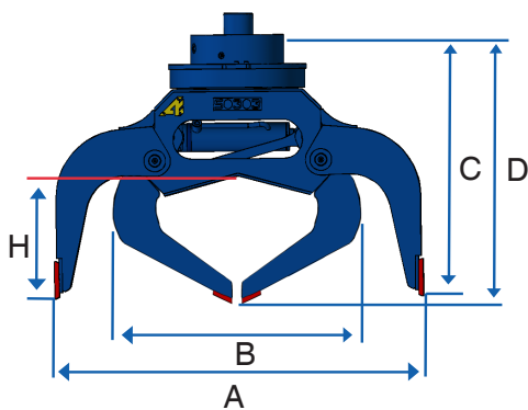
Pohľad na S0223 až S0453
