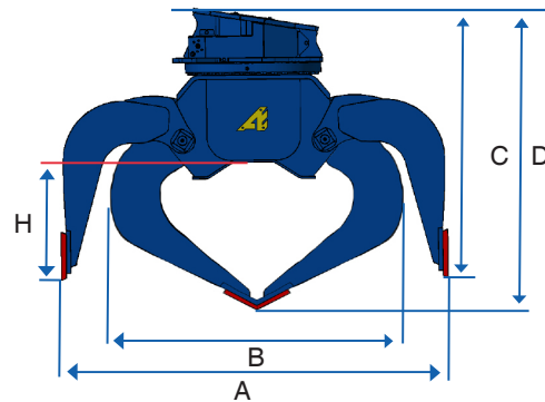
Pohľad na S3002 až S6002
