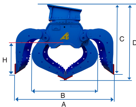
Pohľad na S0604 až S2304***
