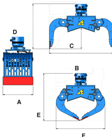
Pohľad na model S180G
