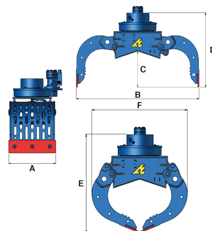
Pohľad na model S250G
