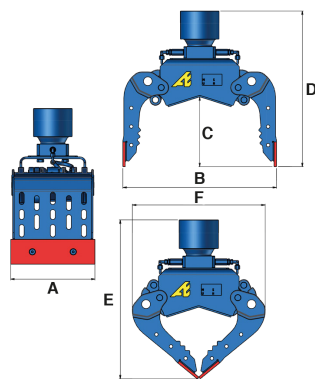
Pohľad na model S080G alebo S100G
