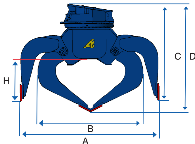
Garras de fondo macizo
